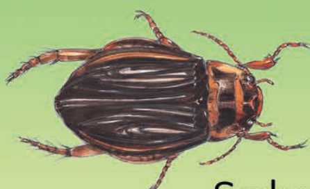
Schwimmkäfer 7-8 mm
