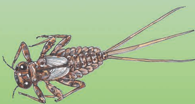
Eintagsfliegenlarve 8-12 mm
