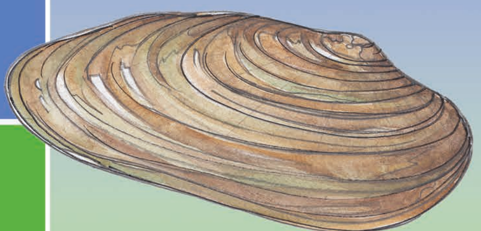
Flussmuschel 60-140 mm
