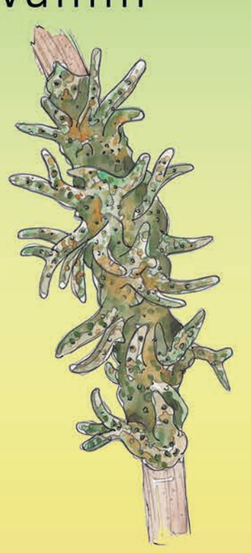
Süßwasserschwamm
