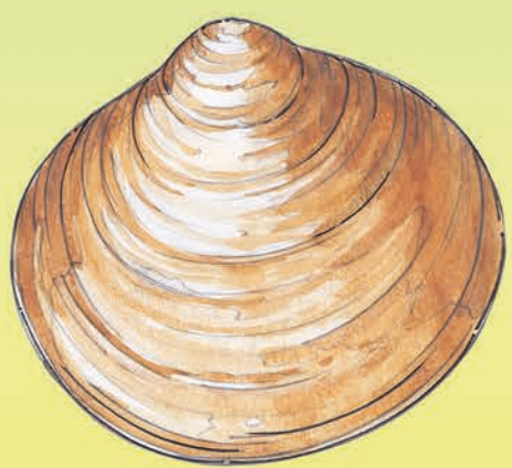
Kugelmuschel 10-14 mm
